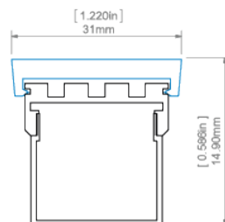
GIZA profile with G-K cover and GIP mounting bracket profil GIZA z oslóną G-K oraz mocowníkem GIP
