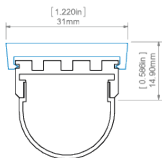
GIZA profile with G-L cover and GIP mounting bracket profil GIZA z oslóną G-L oraz mocowníkem GIP
