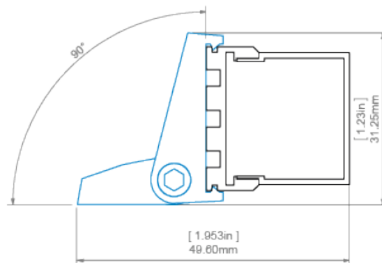
GIZA profile with G-K cover and REGIP-UV mounting bracket profil GIZA z osłoną G-K oraz mocownikiem REGIP-UV
