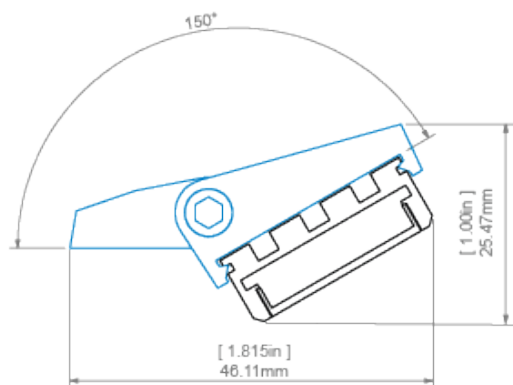
GIZA profile and REGIP-UV mounting bracket profil GIZA z mocovníkem REGIP-UV
